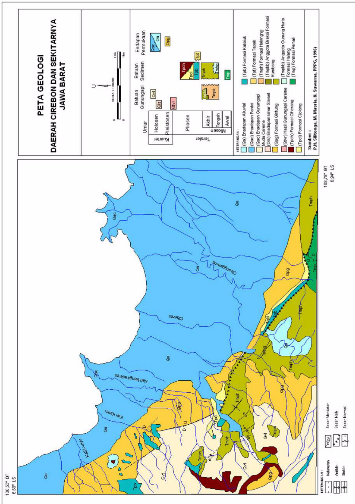
Gambar 2. Peta geologi daerah studi dan sekitarnya (Modifikasi P.H. Silitonga 1996)
