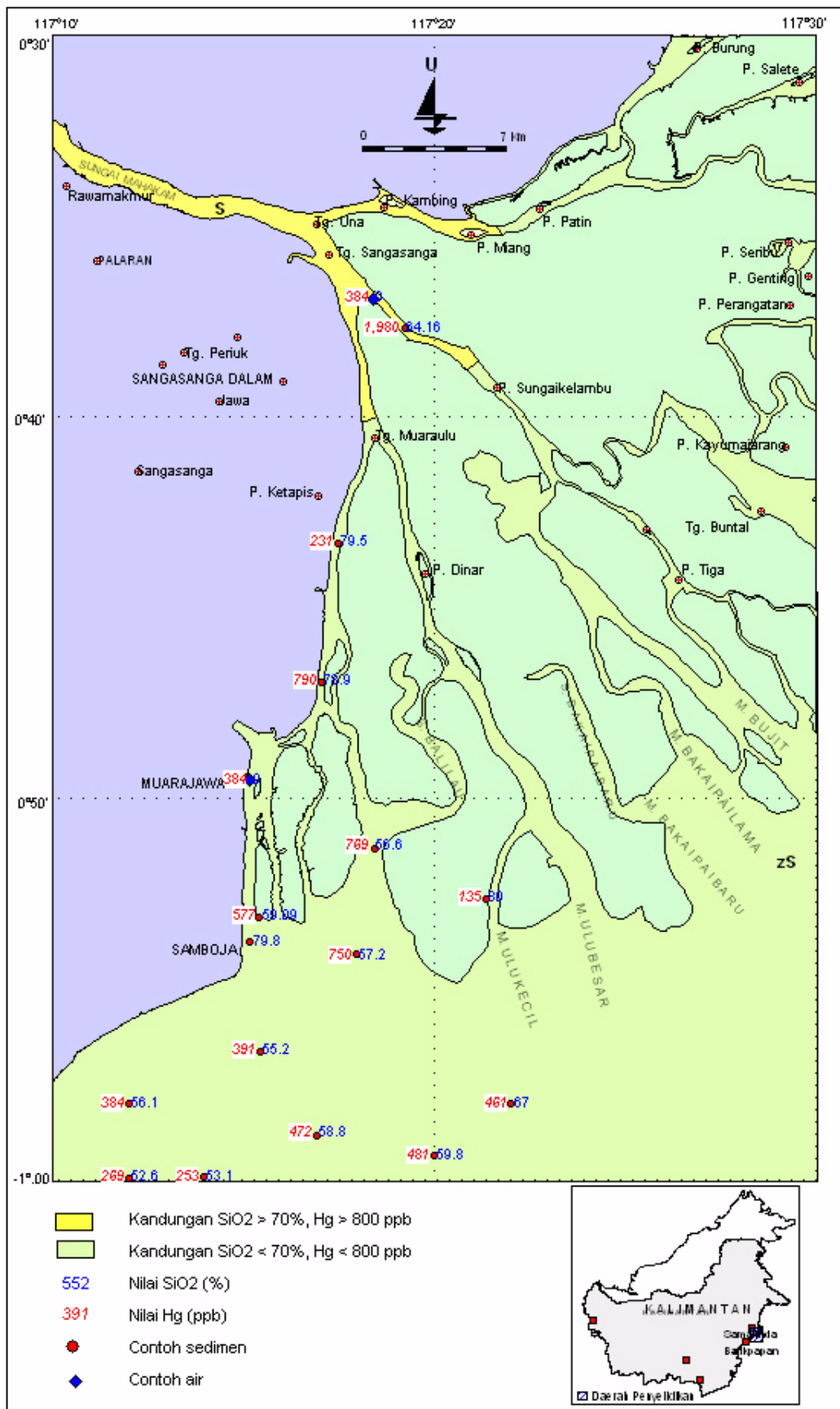
Gambar 2 Peta kandungan unsur utama (SiO 2 ) dalam % dan Hg (ppb) pada sedimen permukaan dan contoh air, perairan Delta Mahakam
