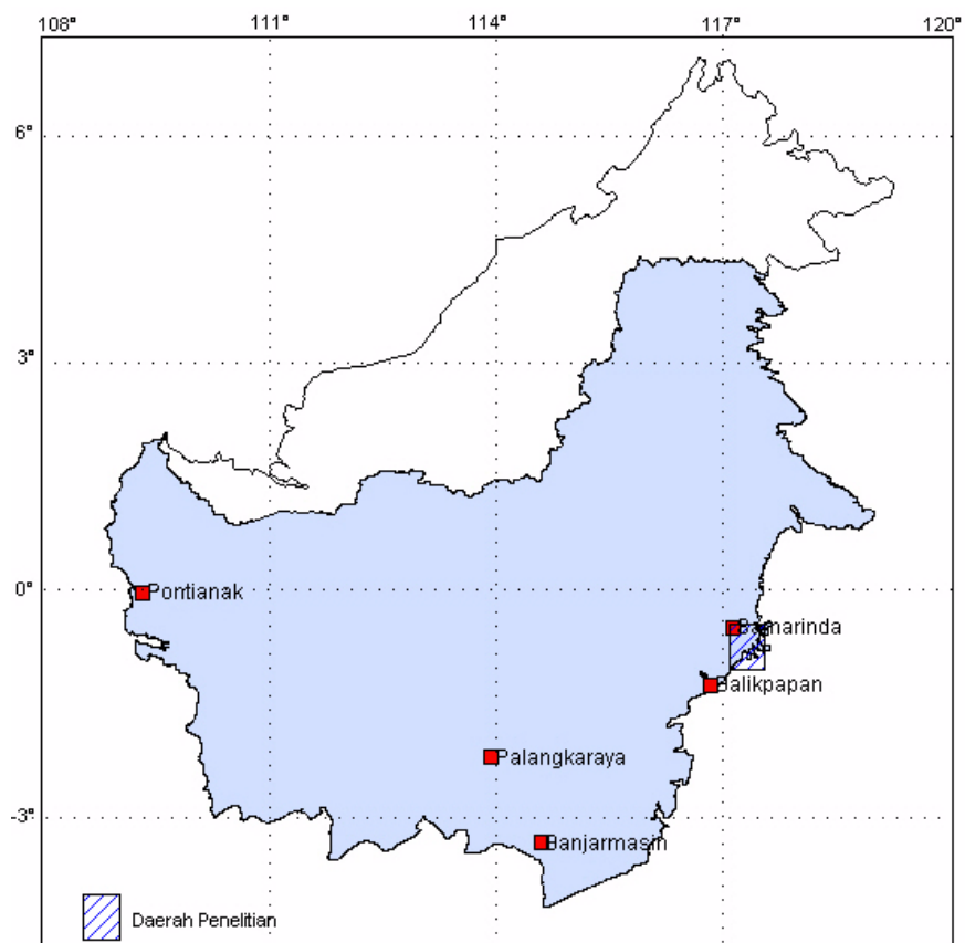
Gambar 1 Peta lokasi daerah penelitian, perairan Delta Mahakam Kalimantan Timur
