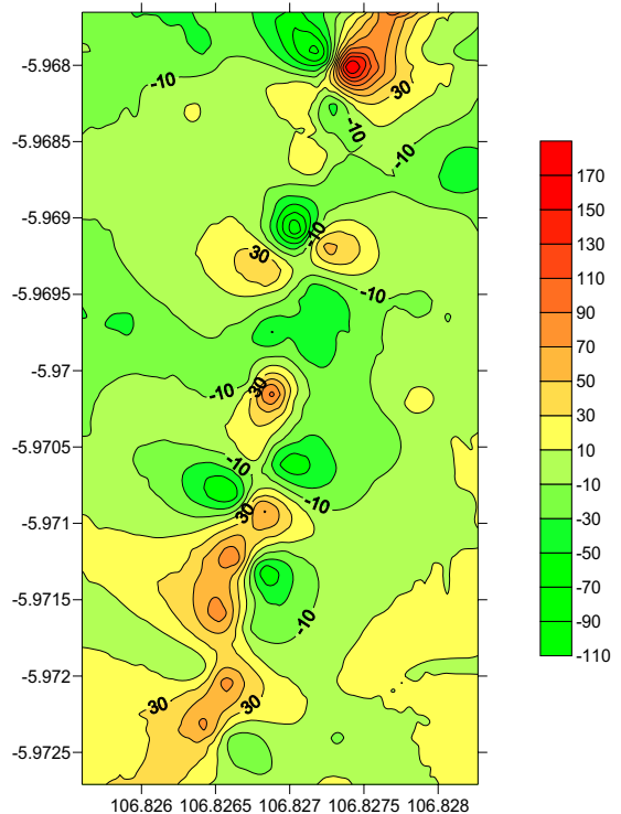
Gambar 3. Peta Anomali Magnet dengan penerapan RTP 2D menggunakan Matlab
