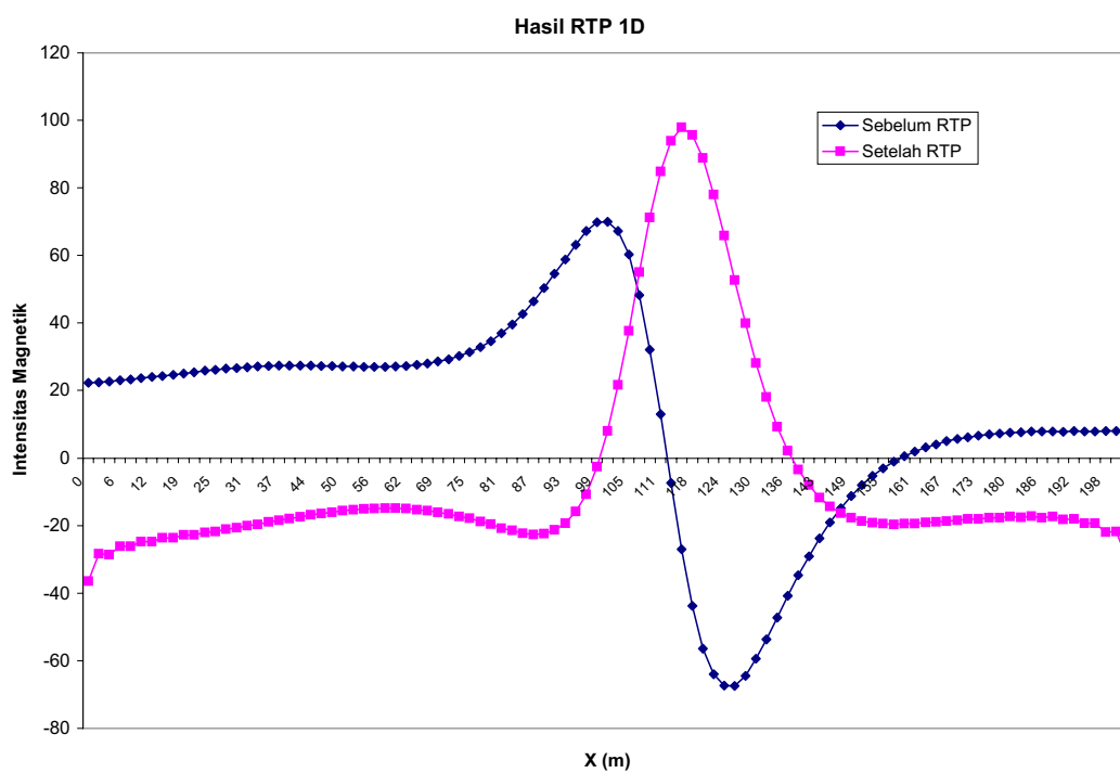
Gambar 6. Kurva perbandingan data sebelum dan setelah RTP
