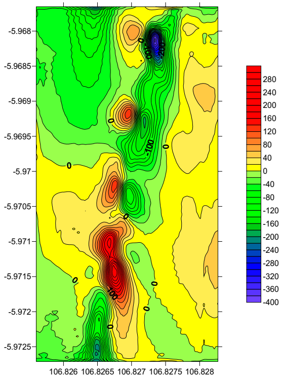
Gambar 4. Peta Anomali Magnet dengan penerapan RTP 3D menggunakan Matlab
