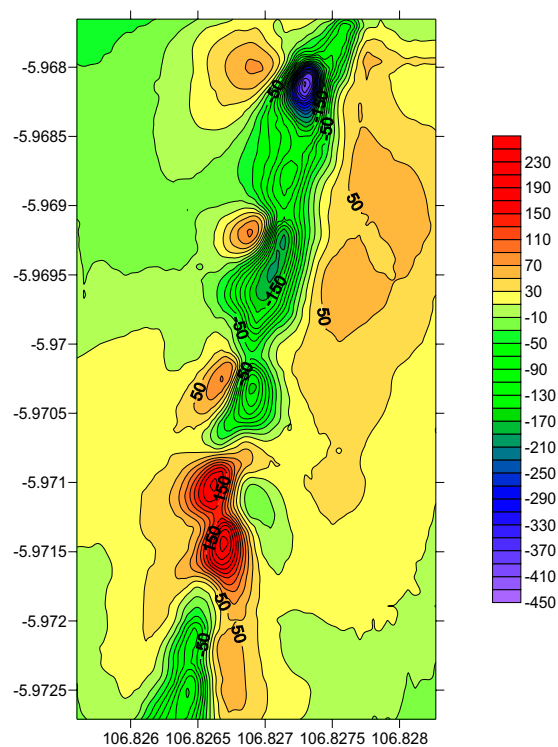
Gambar 5. Peta Anomali Magnet dengan penerapan RTP 3D menggunakan Magpick
