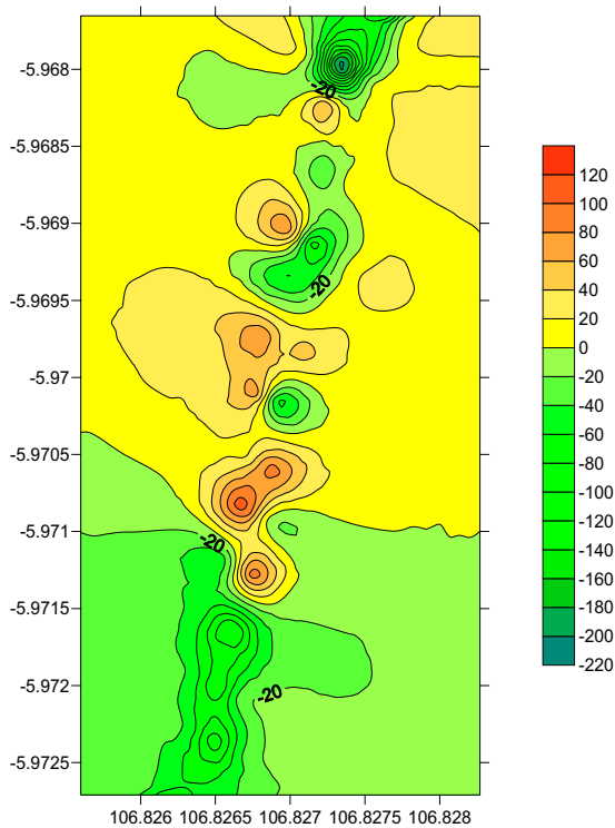
Gambar 2. Peta Anomali Magnet Total sebelum penerapan RTP (gridding dilakukan dengan surfer)
